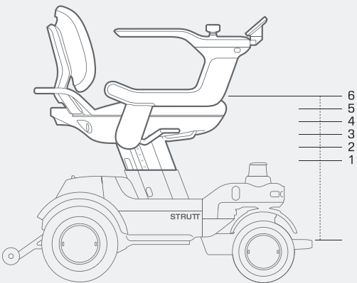
座椅高度
